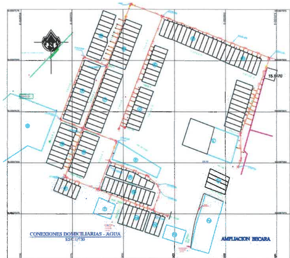
Planta de conexiones domiciliarias de agua potable.
