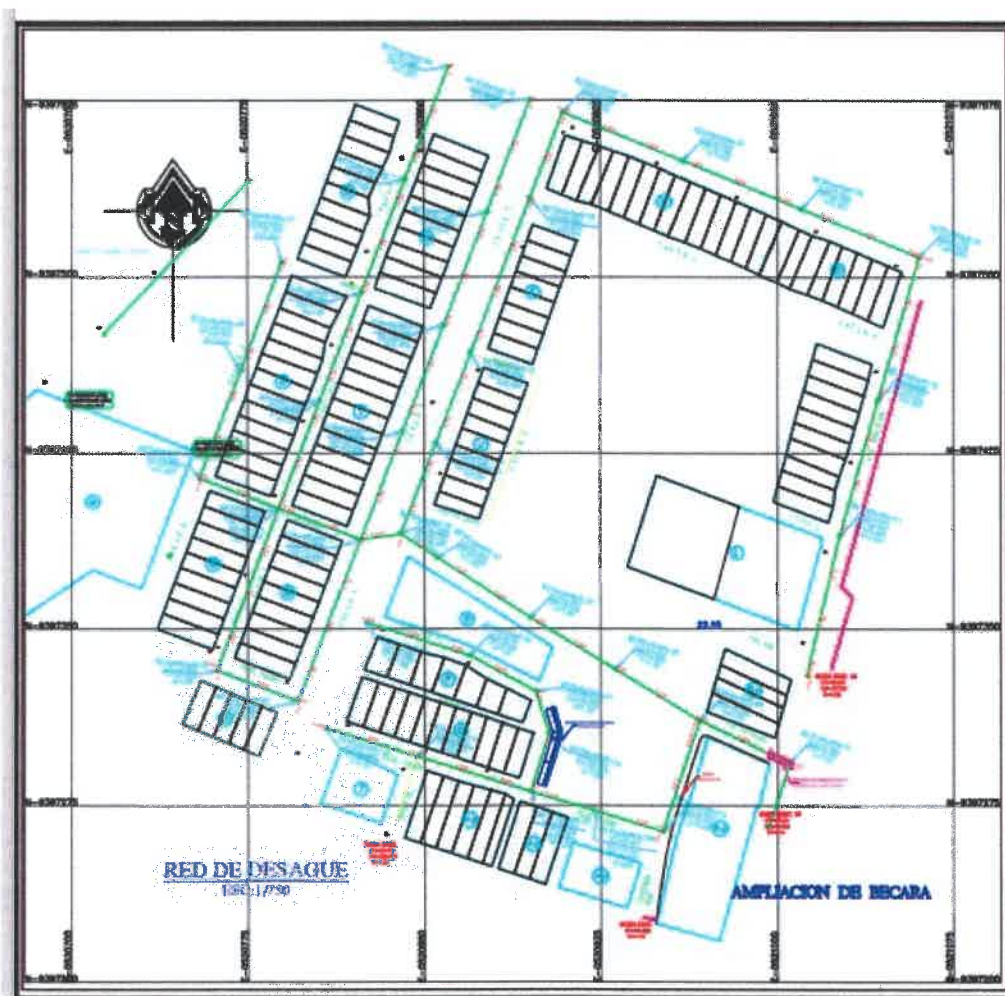
Planta general de la red colectora.
