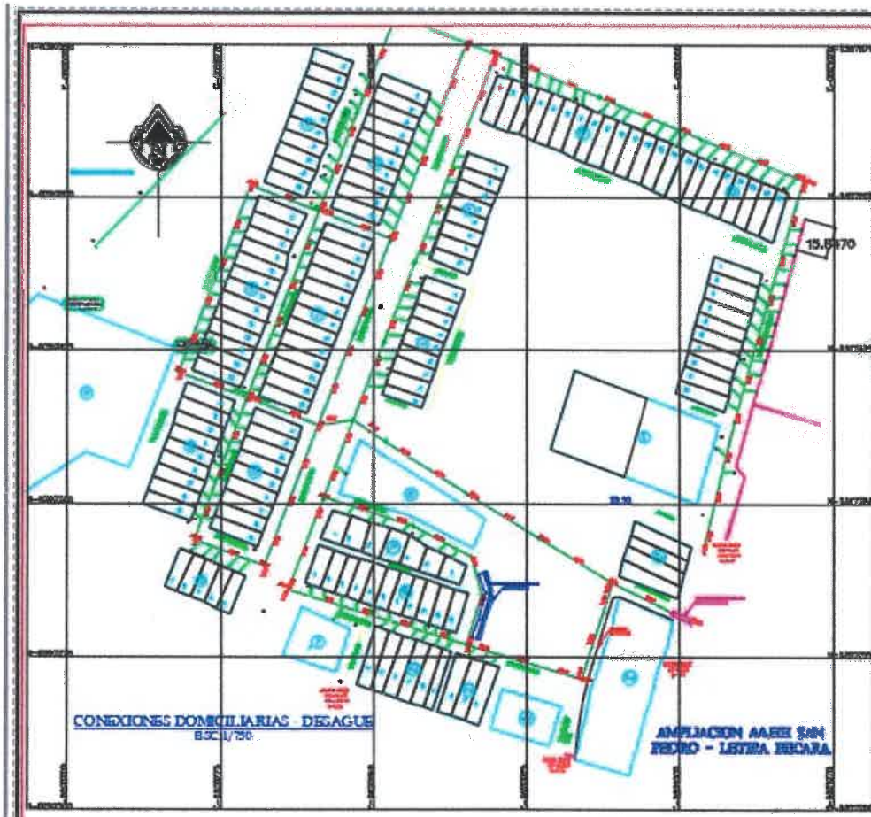
Planta conexiones domiciliarias de desagüe.
