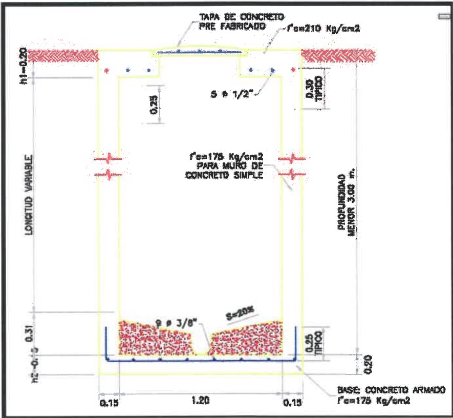
Detalle buzón típico I.
