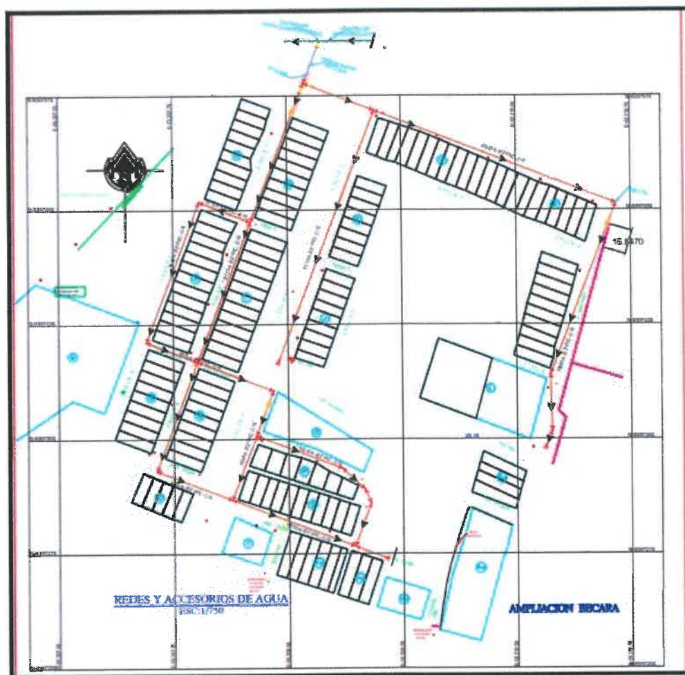
Planta redes de distribución de agua potable.
