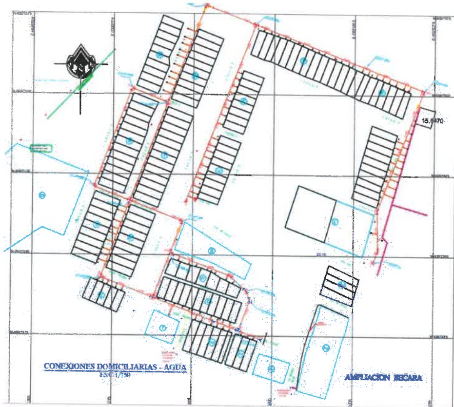
Planta de conexiones domiciliarias de agua potable.
