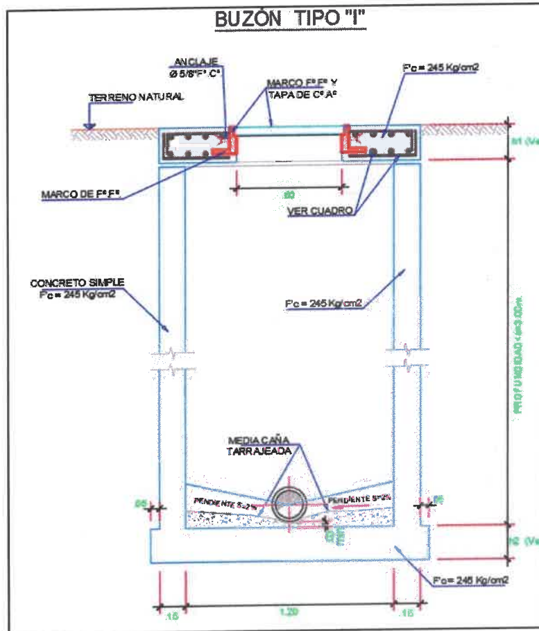
Detalle buzón típico I.
