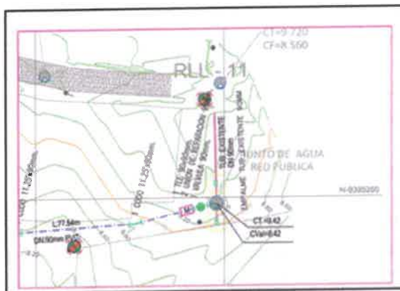
Punto de empalme de agua potable en la red existente
