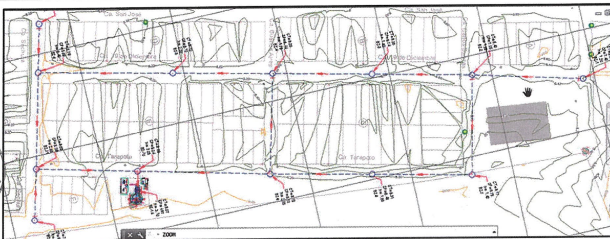
Planta general de la red colectora.
