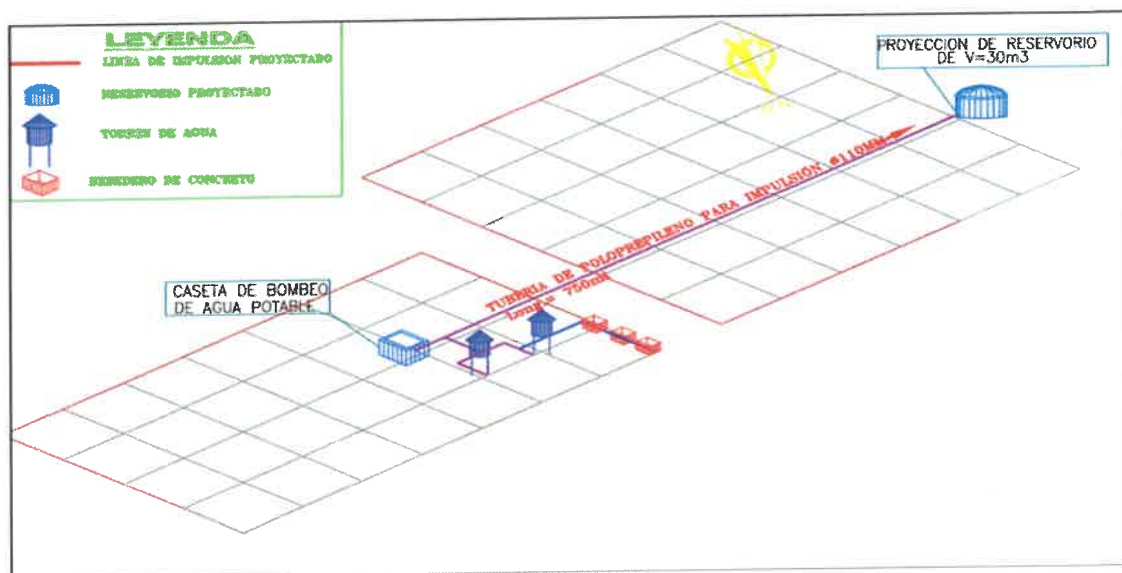
Figura N°03: Isométrico de la Planta General del proyecto.
