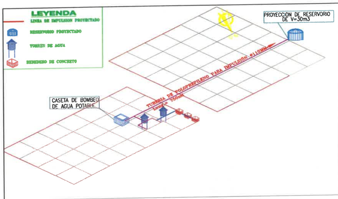
Figura N°03: Isométrico de la Planta General del proyecto.
