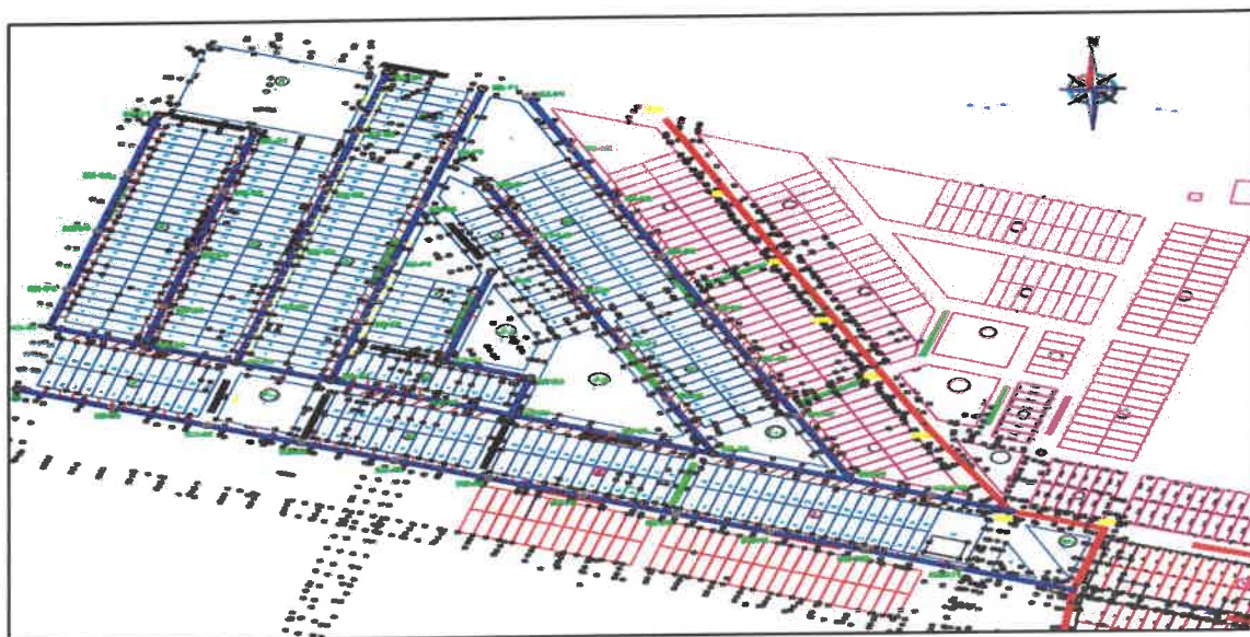
Planta conexiones domiciliarias de desagüe.
