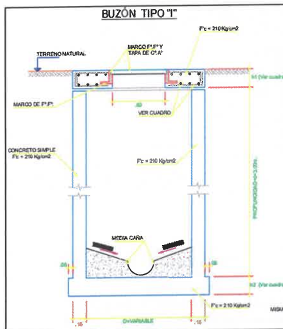
Detalle buzón típico I.
