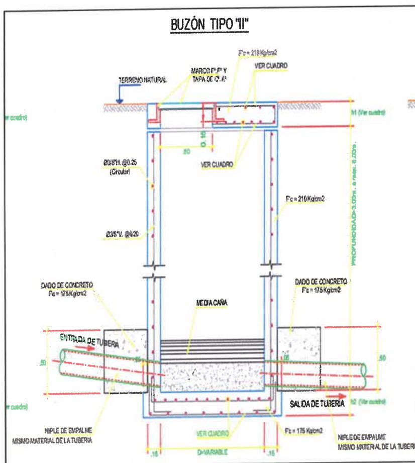
Detalle buzón típico II.
