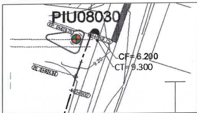
Cotas de buzón receptor o de empalme
