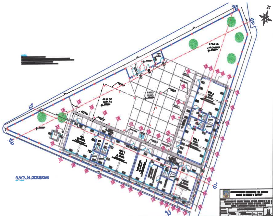
Figura N°03: Planta General del proyecto
