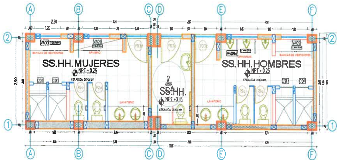
MODULO 2 - SS.HH. PUBLICO PARA ÁREA DEPORTIVA
