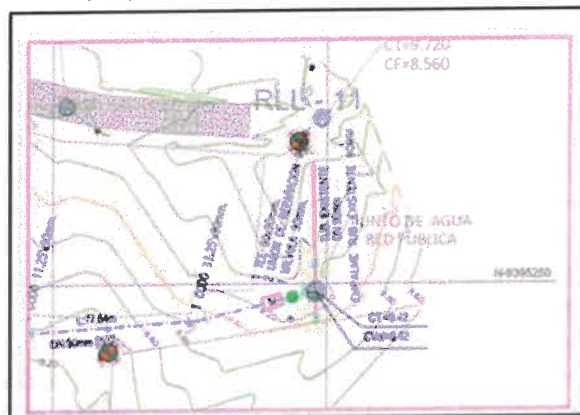
Punto de empalme de agua potable en la red existente
