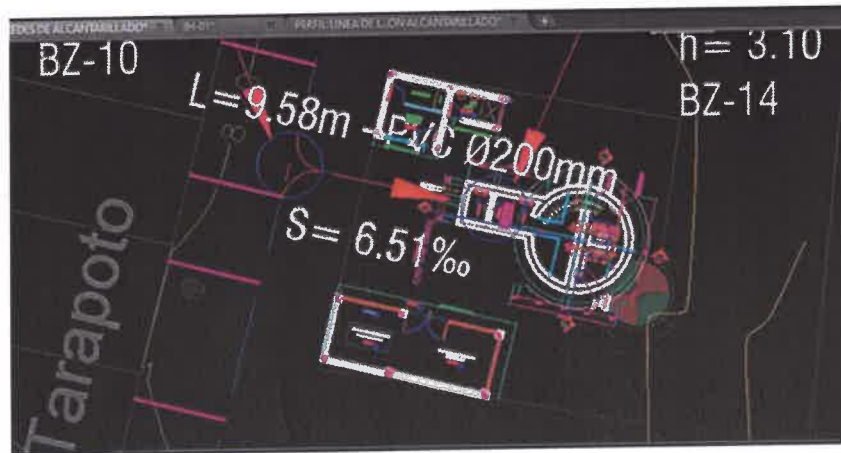
Cámara de bombeo de aguas residuales.
