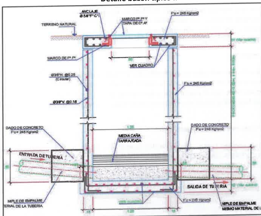
Detalle buzón típico I.
