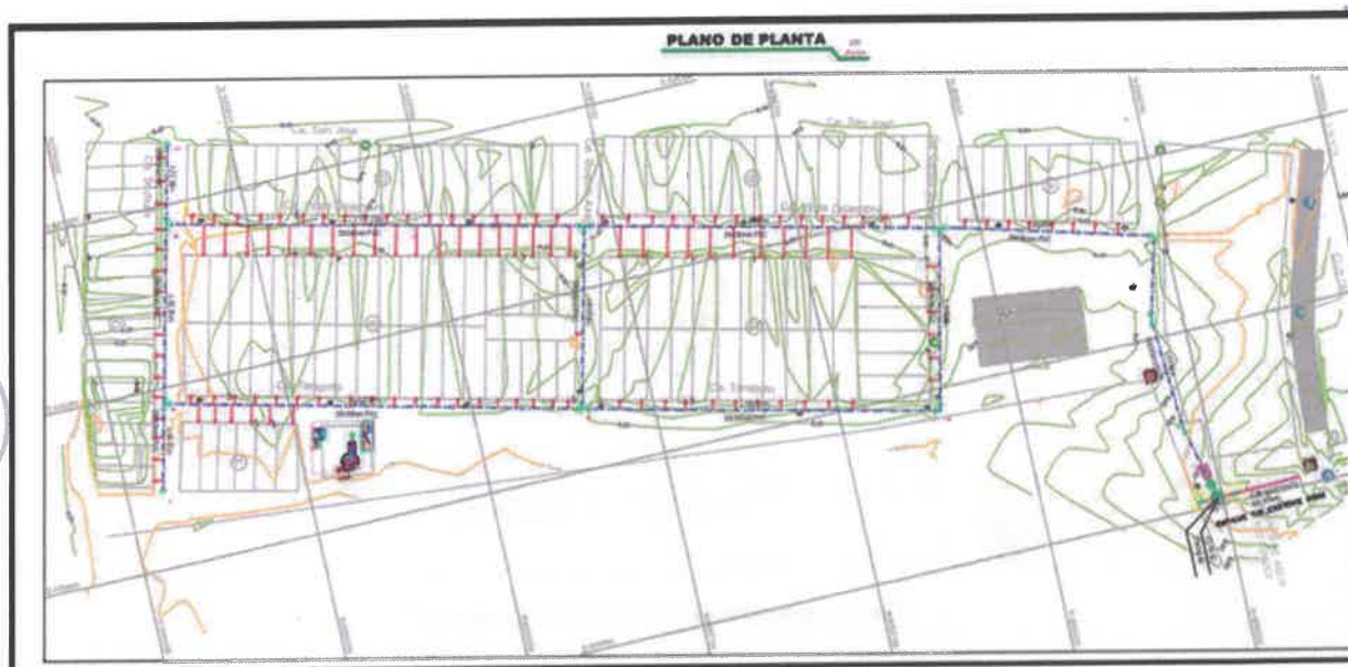
Planta de conexiones domiciliarias de agua potable.
