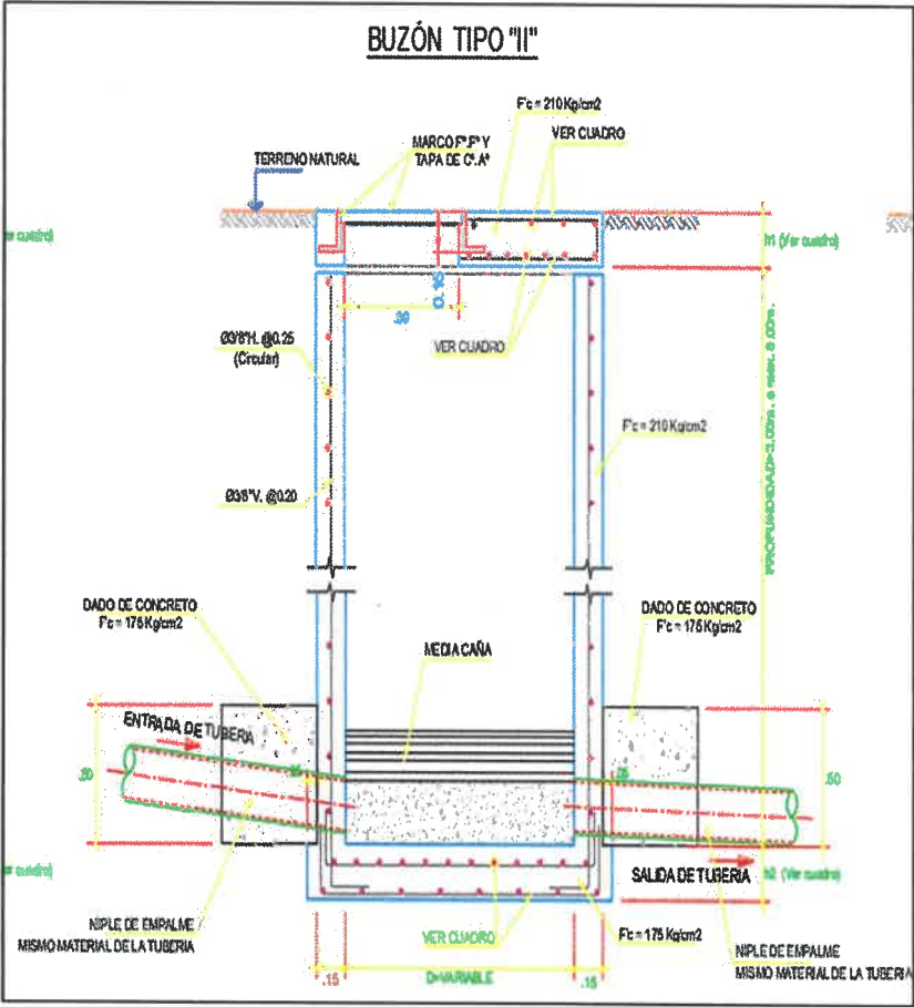
Detalle buzón típico II.
