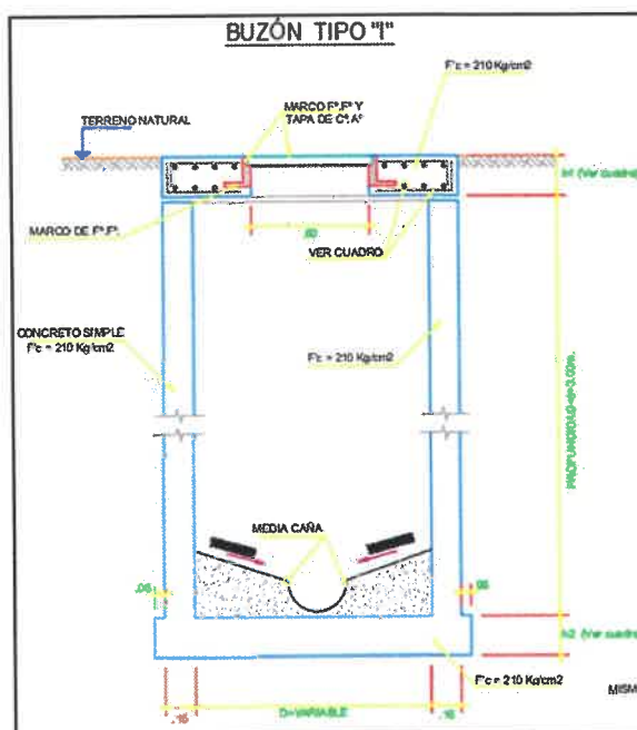
Detalle buzón típico I.
