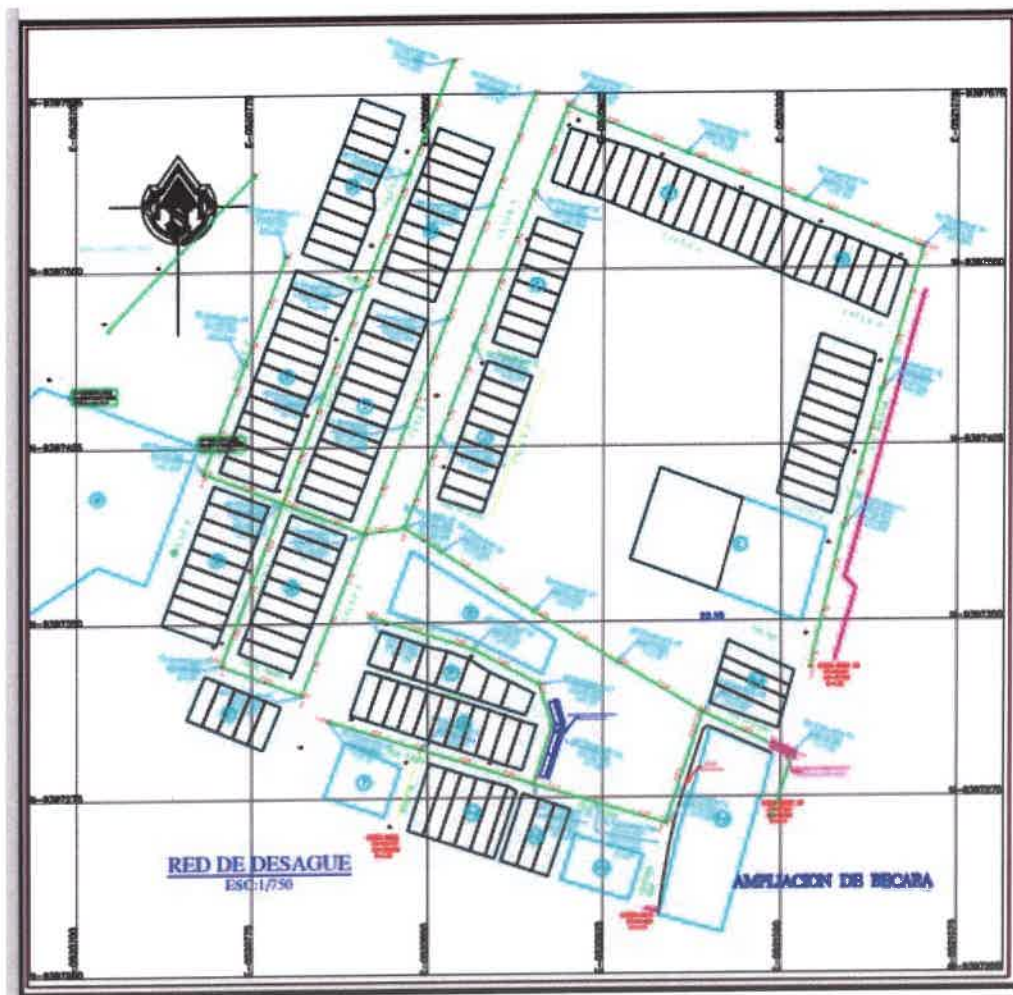
Planta general de la red colectora.
