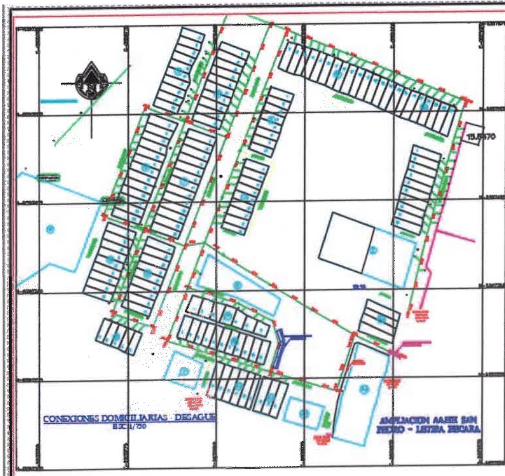
Planta conexiones domiciliarias de desagüe.
