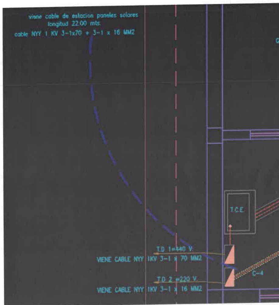
Figura N° 04. Es correspondencia del contratista implementar los tableros eléctricos. La conexión a la alimentación eléctrica será correspondencia de El contratista del Componente 02, el mismo que deberá realizar las pruebas de puesta en marcha y programación correspondiente, de acuerdo con las cargas requeridas por los equipos.
